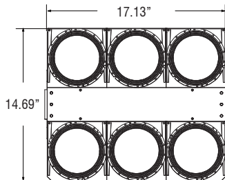
420W / 6 Modules
